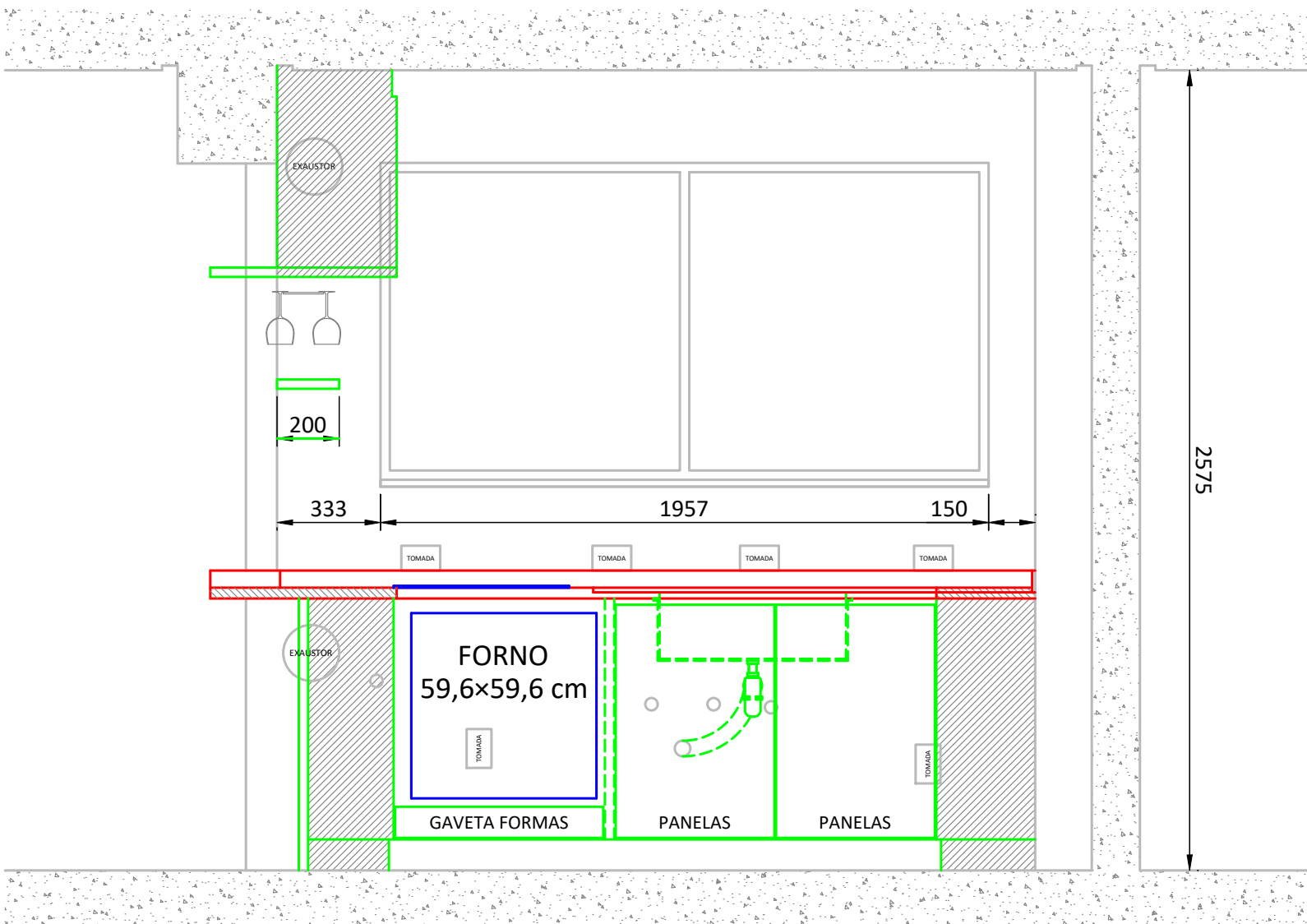
CORTE AA
