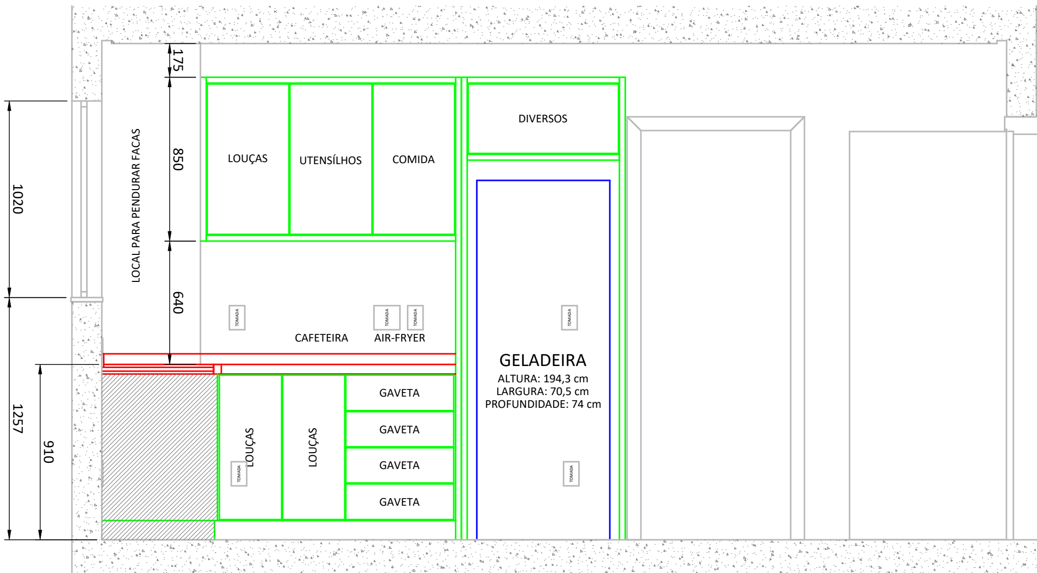
CORTE BB
